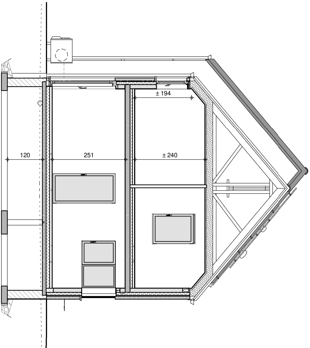
COUPE AA
