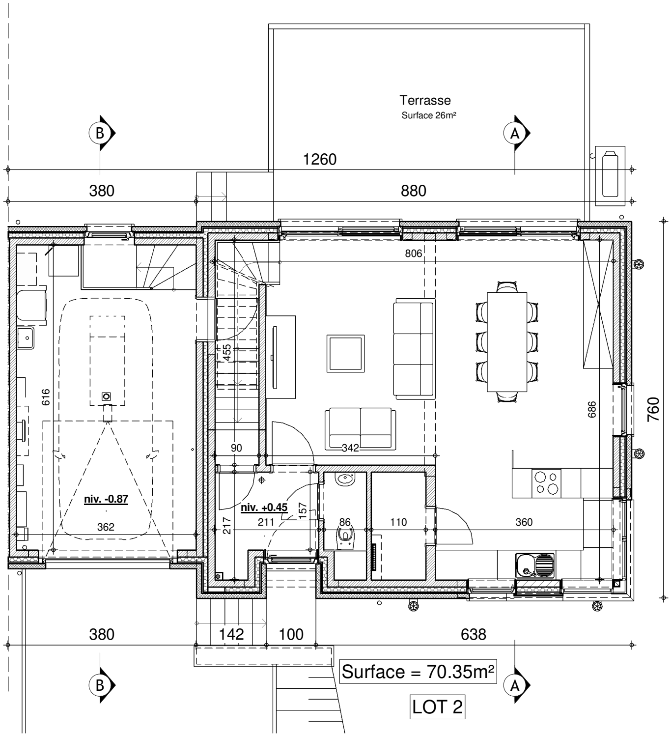
REZ-DE-CHAUSSEE
