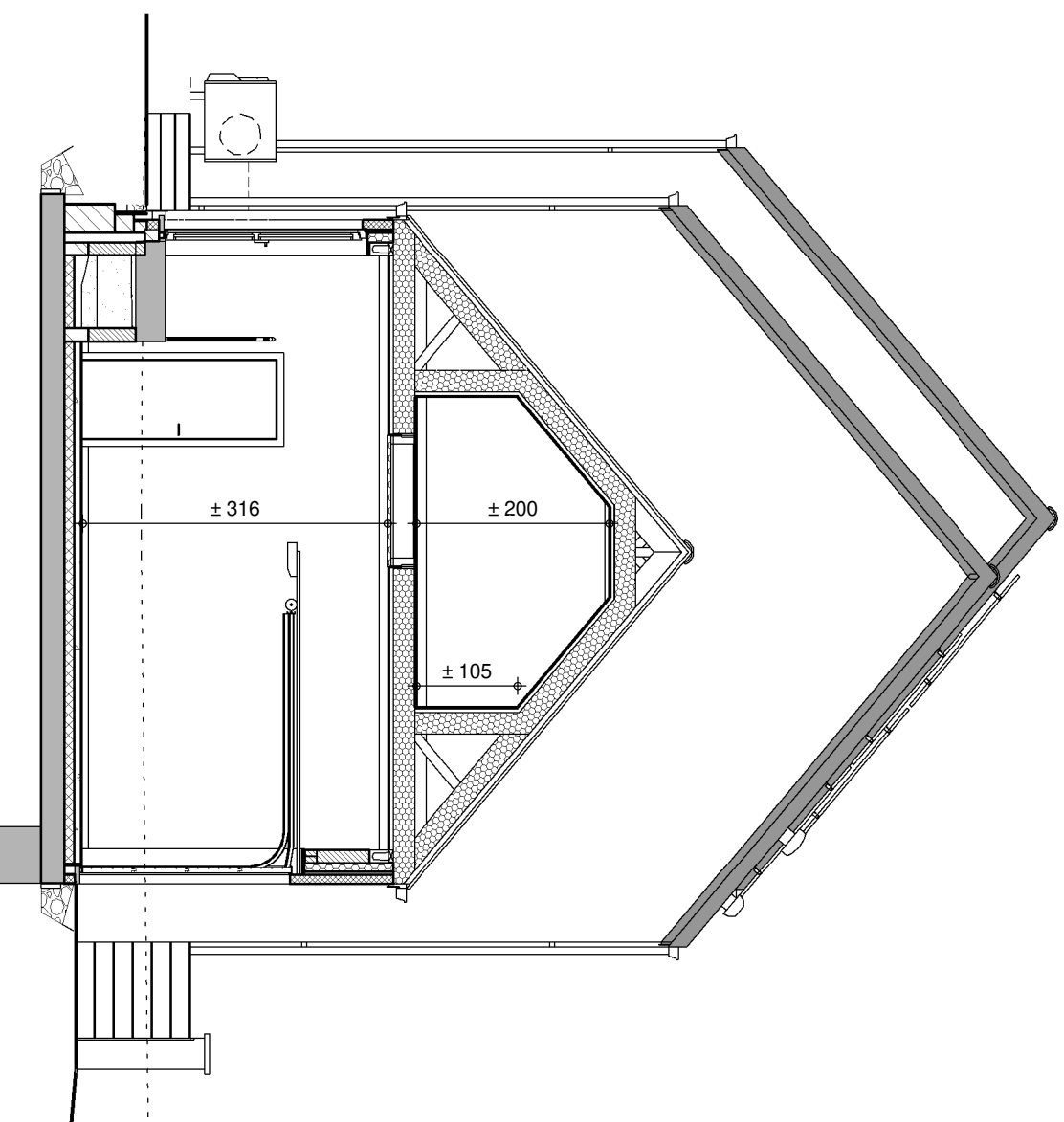
COUPE BB
